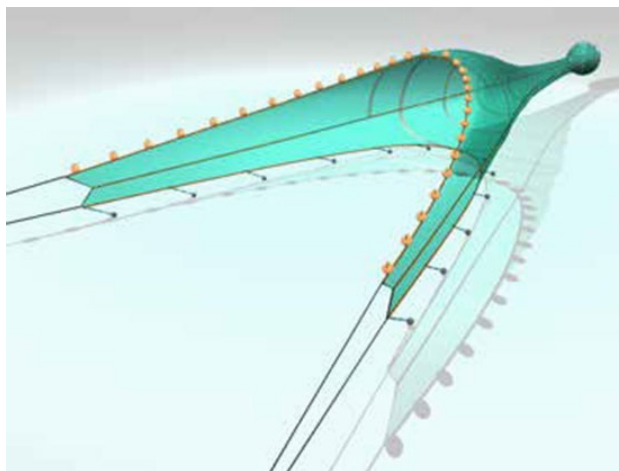
Figur 6.1.4. Trawl med dropkæder fæstnet til undertællen som erstatning for ruppen, der trækkes hen over bunden.
