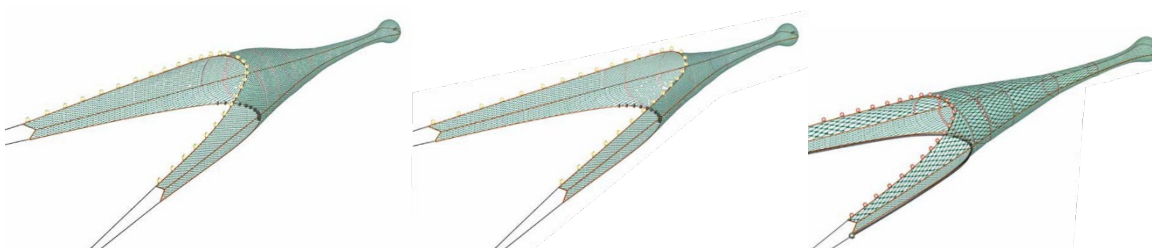
Figur 6.1.6. En standard-bundtrawl til fisk sammenlignet med en topløs trawl og en trawl med store masker i taget. Begge ændringer vil føre til en reduktion af den hydrodynamiske slæbemodstand.
