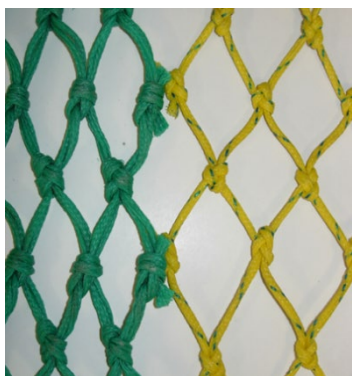
Figur 6.1.5. To netstykker med samme maskestørrelse, men fremstillet af hhv. dobbelt- og enkeltråd demonstrerer, hvordan et redskabs hydrodynamiske slæbemodstand kan reduceres uden tilpasning af maskestørrelsen.
